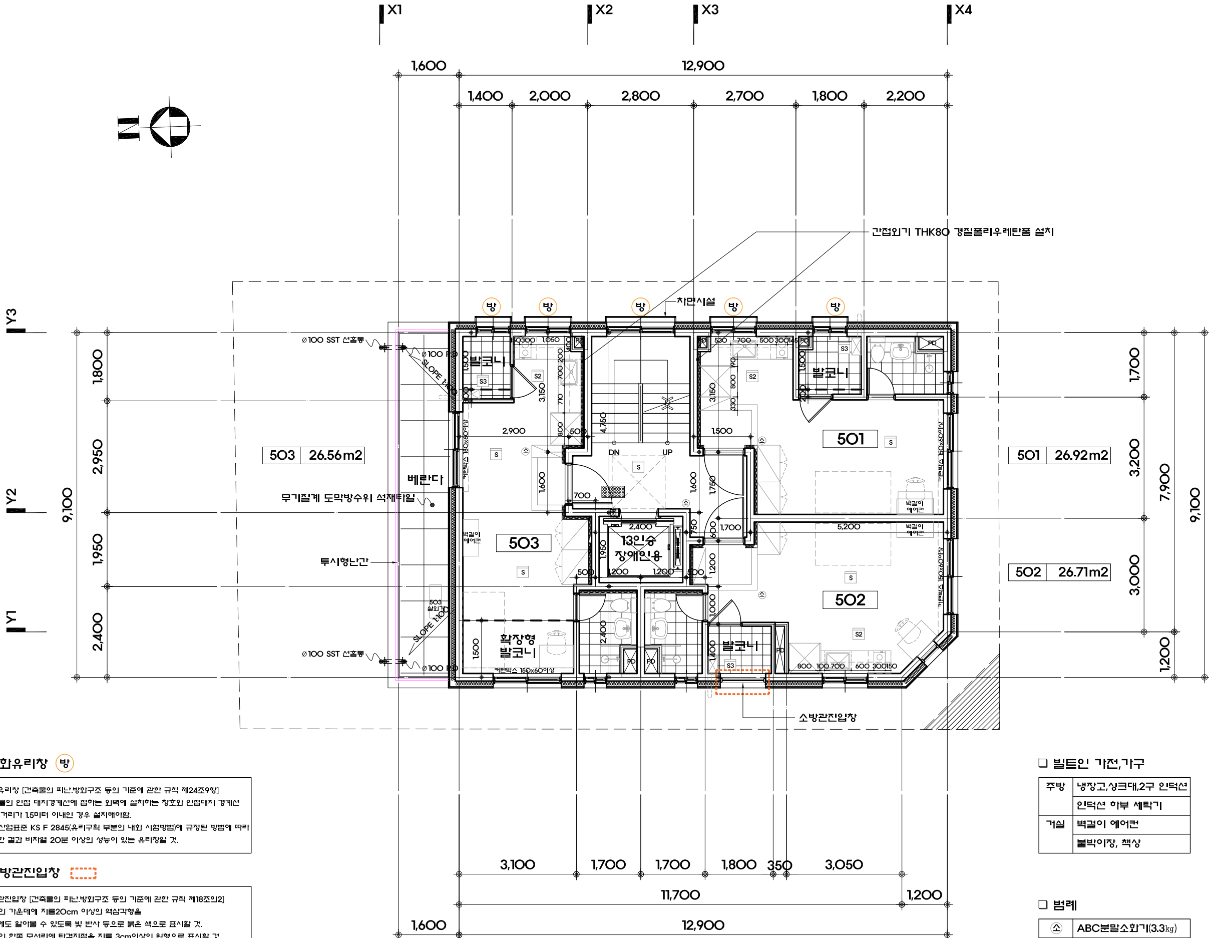
지상 5층 평면도 축척 : 1/100
